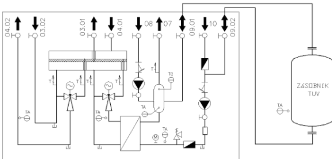
Obr. č. 4 Blok ohřevu užitkové vody (voda - voda) s jednou přiřazenou otopnou sekcí Regulace výkonu ejektory
