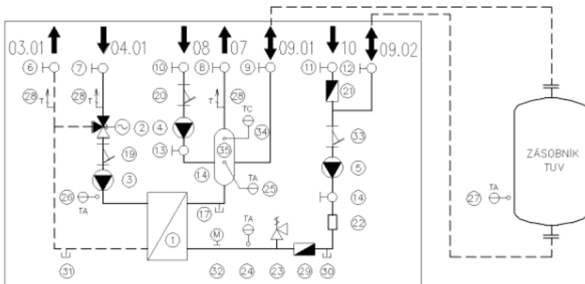
Obr. č. 1 Blok ohřevu užitkové vody (voda - voda) Regulace výkonu směšovacím čerpadlem
