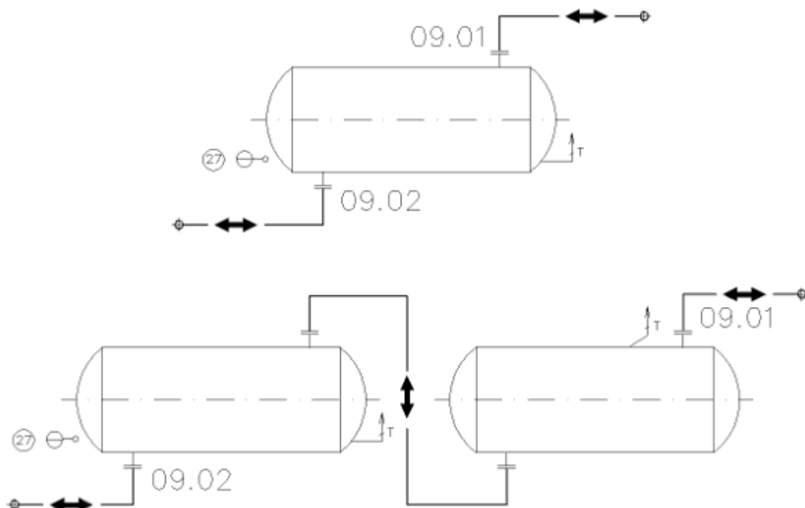
Obr. č. 6 Připojení ležatých zásobníků užitkové vody
