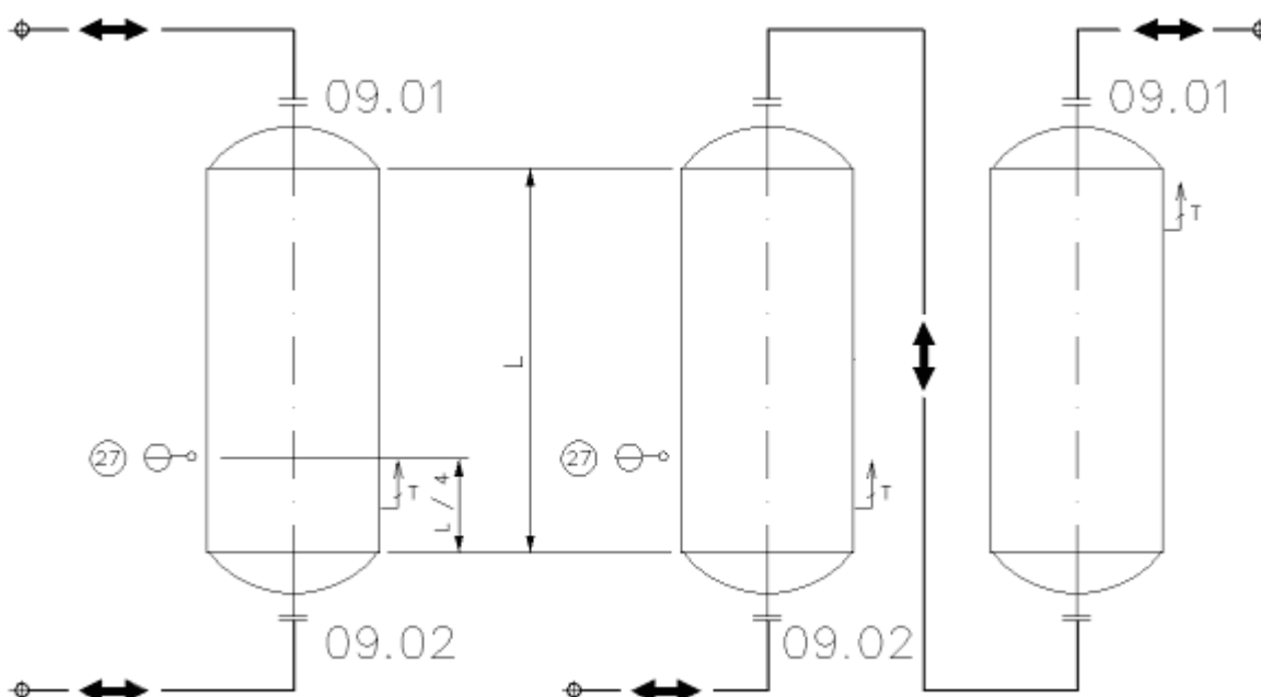
Obr. č. 5 Připojování stojatých zásobníků užitkové vody
