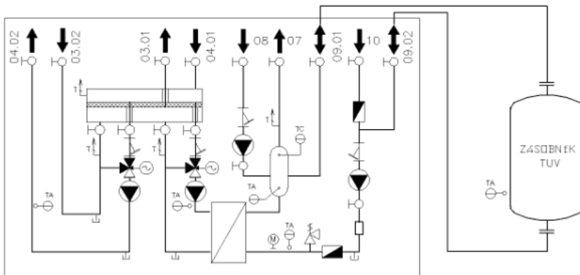
Obr. č. 3 Blok ohřevu užitkové vody (voda - voda) s jednou přiřazenou otopnou sekcí Regulace výkonu směšovacími čerpadly
