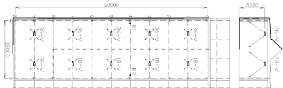
Obr. 2 - Půdorys a řez objektu vytápěného světlými infrazářiči, krajní loď - u venkovních stěn zářiče vyšších výkonů
