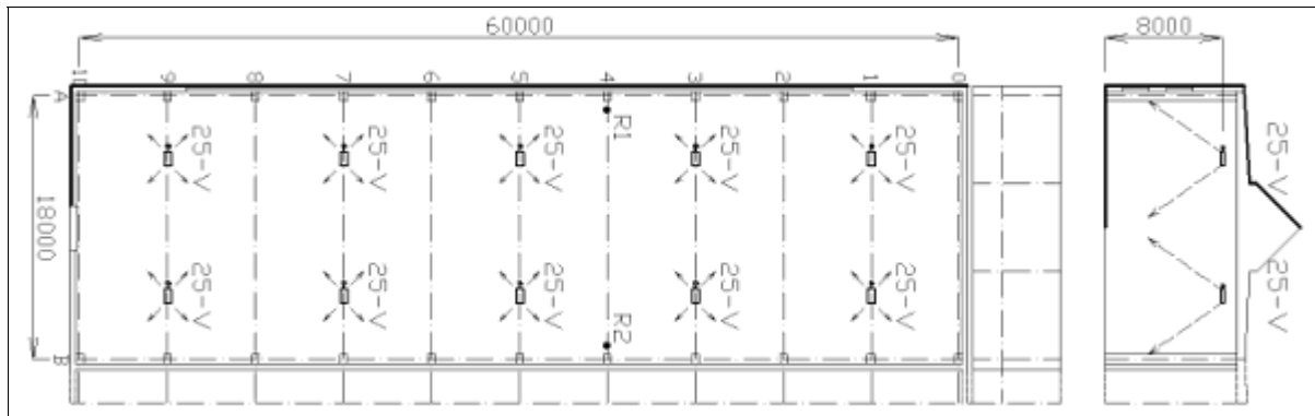
Obr. 1 - Půdorys a řez objektu vytápěného světlými infrazářiči, krajní loď - zářiče stejného výkonu
