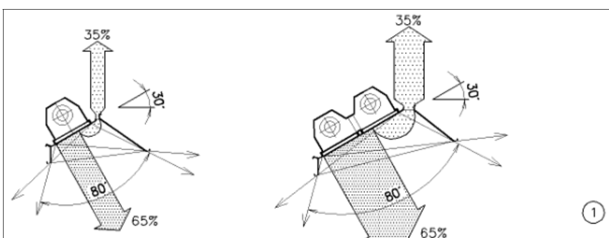
Obr. 1 - Světlé zářiče se speciálně upravenými reflexními zářivkami pro vytápění osamělých pracovišť
