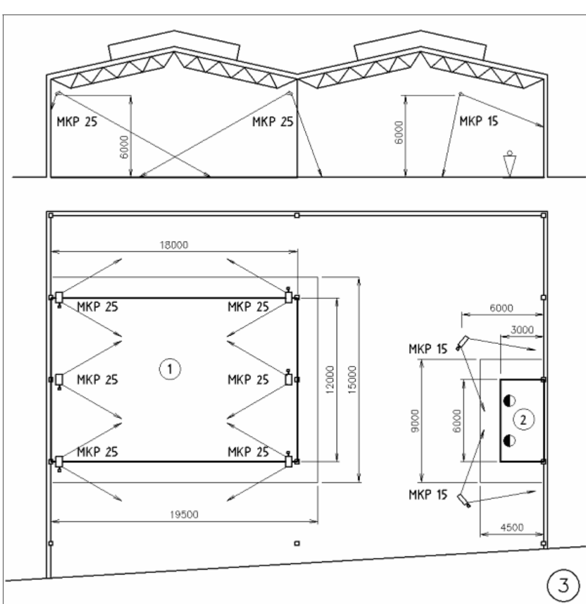
Obr. 3 - Vytápění osamělých pracovišť v nevytápěné hale 1 - plocha 12 x 18 m = jedno pole haly; 2 - pracoviště u okna 6 x 3 m
