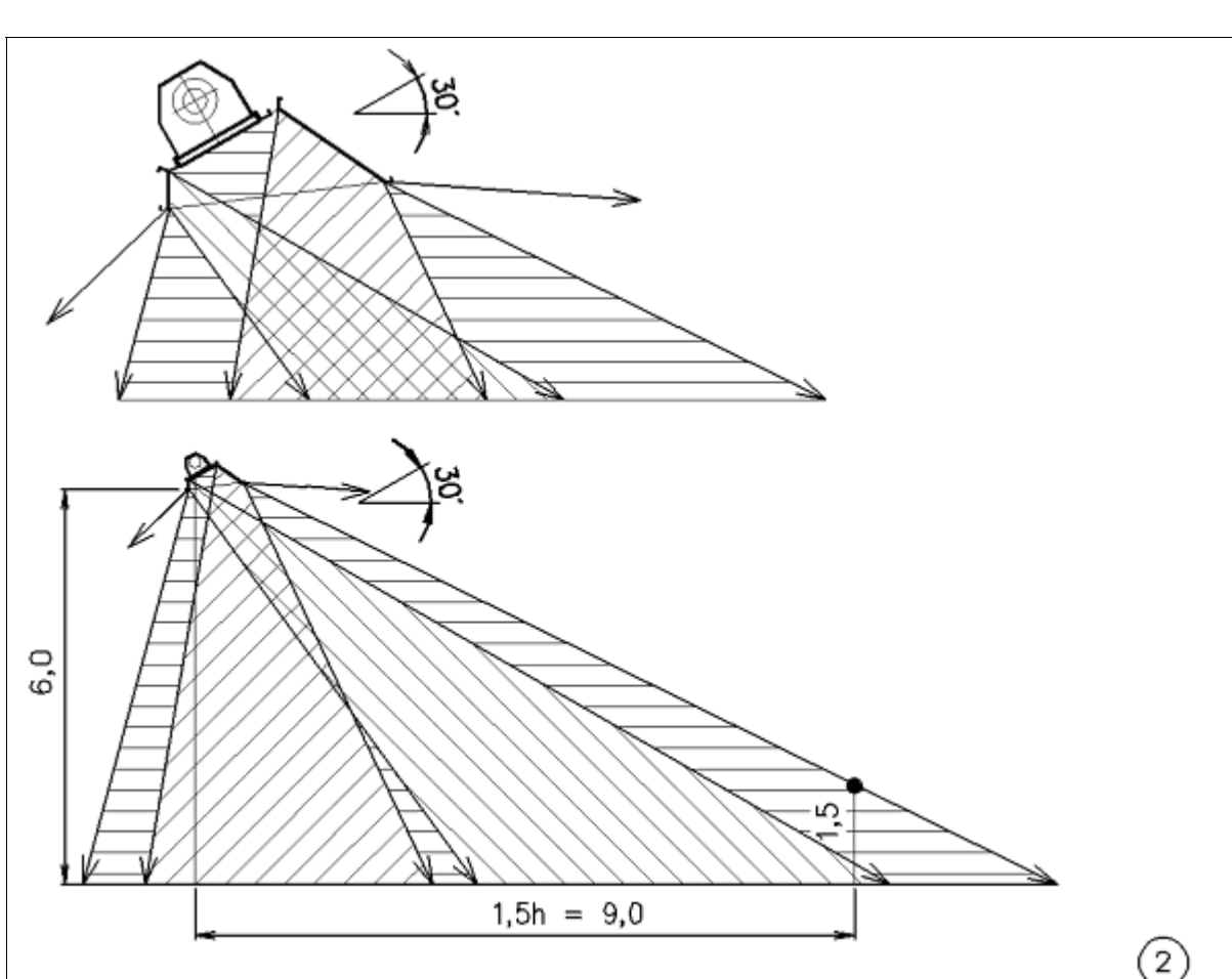
Obr. 2 - Světly zářič - koncentrování toku tepelné energie sáláním
